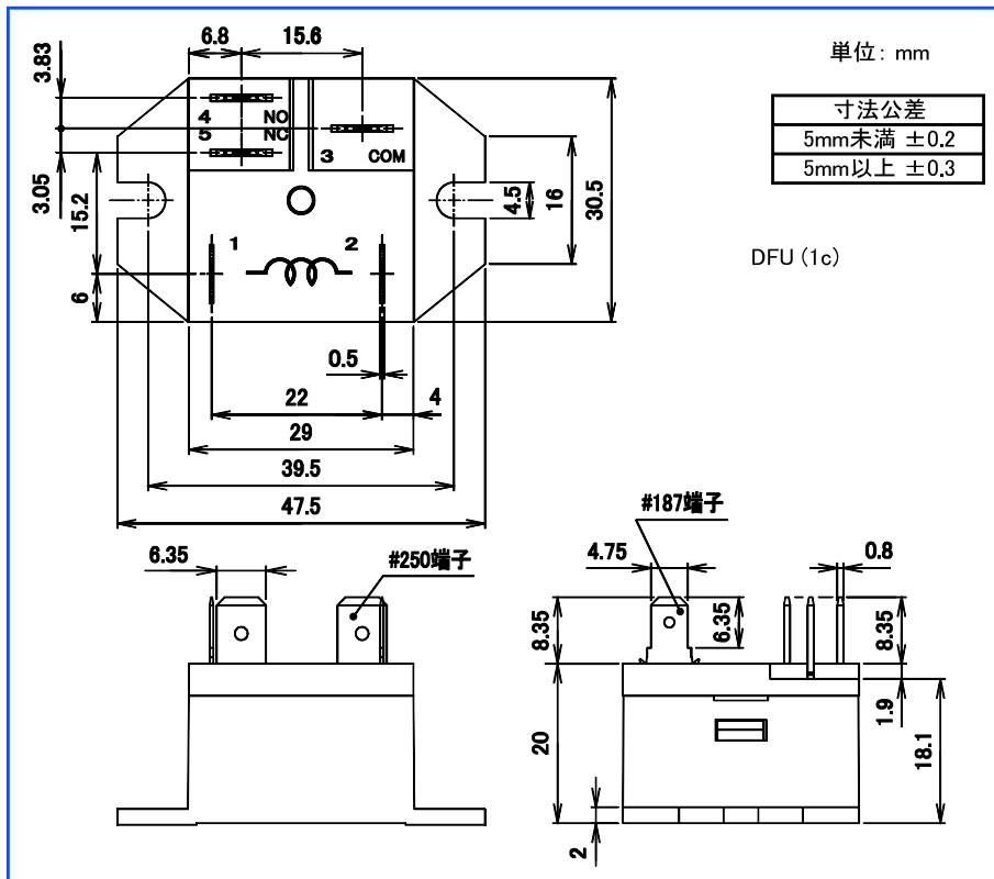
■ 外形寸法図
